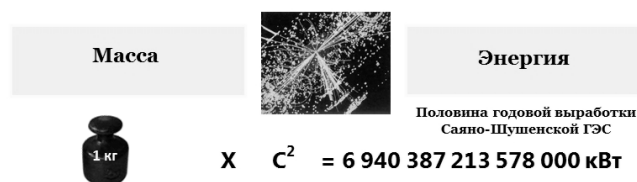
Рис. 10. Бозонный уровень энергии
